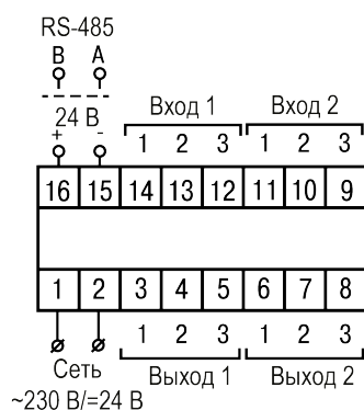
Рисунок 5.5 – Общая схема подключения TRM12–Щ5
