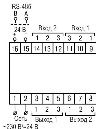
Рисунок 5.6 – Общая схема подключения TRM12–Д
