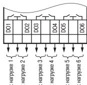
Рисунок 9 – Схема подключения ВЭ типа «Р»
