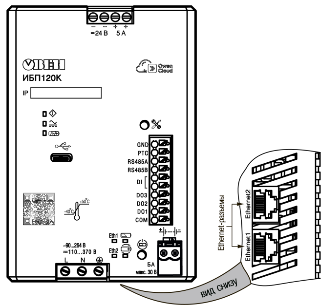
Рисунок 6.7 – Лицевая панель прибора
