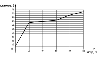
Рисунок 6.2 – График заряда током 2,6 А
