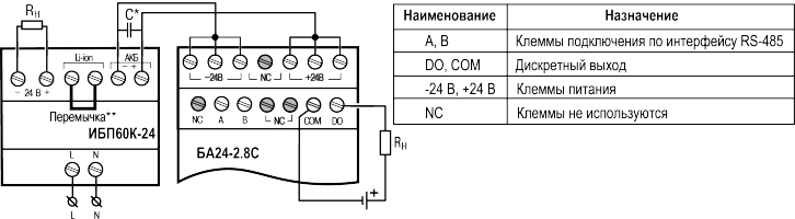
Рисунок 5.1 – Схема подключения
