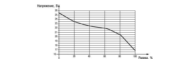
Рисунок 6.3 – График разряда током 3,6 А
