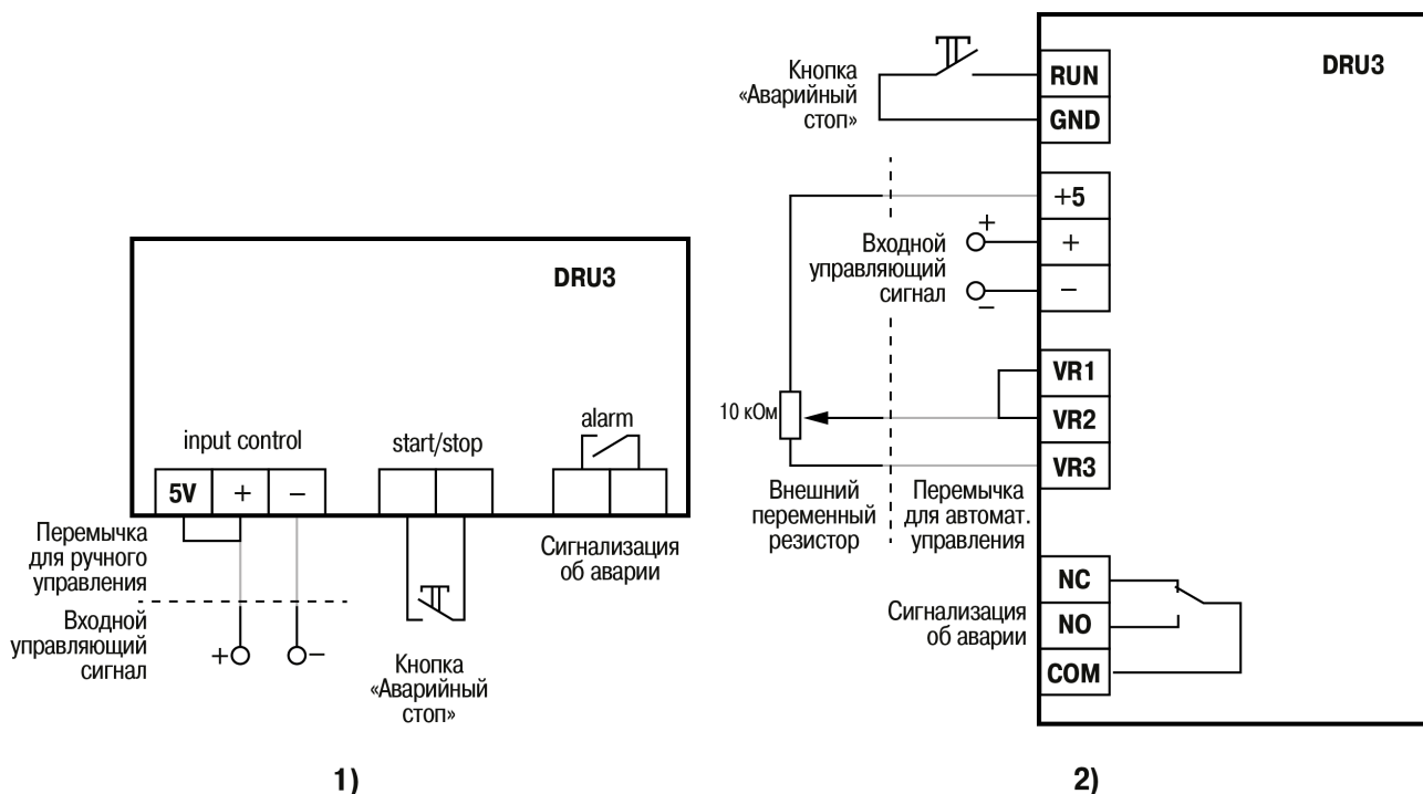
Рисунок 6.3 – Схема подключения сигнальных клемм: (1) DRU3-25/40/75/100; (2) DRU3-125/150/200
