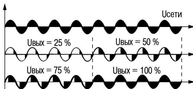
Рисунок 3.4 – Регулировка напряжения
