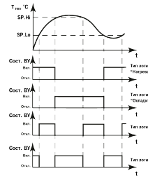
Рисунок 8.1 – Типы логики работы прибора
