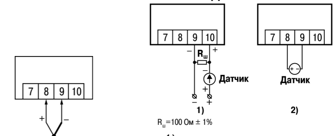
Рисунок 7 – Схема подключения ТП
