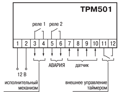
Рисунок 4 – Контакты клеммника
