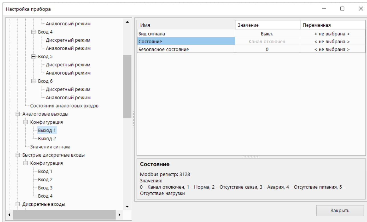
Рисунок 4.15 – Настройка универсальных аналоговых выходов
