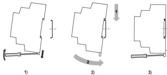
Рисунок 1 – Монтаж прибора
