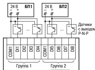
Рисунок 7 – Схема подключения к дискретным входам трехпроводных дискретных датчиков, имеющих выходной транзистор р-р-р-типа с открытым коллектором для сигналов 24 В
