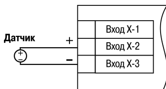
Рисунок 5.14 – Схема подключения активного датчика с выходом в виде напряжения -50...+50 мВ или 0...1 В
