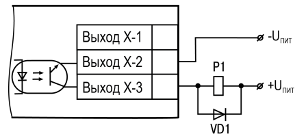
Рисунок 5.20 – Схема подключения нагрузки к ВУ типа «К»
