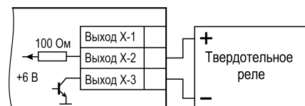
Рисунок 5.21 – Схема подключения нагрузки к ВУ типа «Т»
