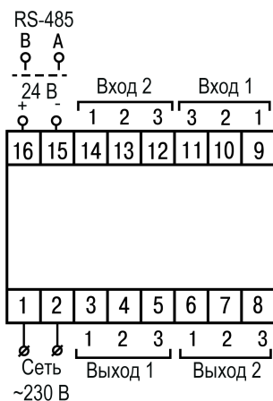
Рисунок 5.6 – Общая схема подключения TPM12–Д
