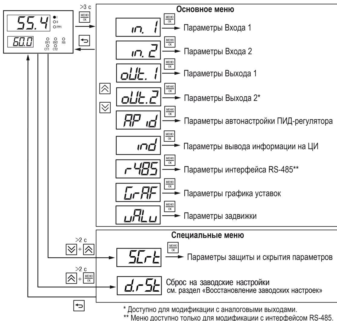
Рисунок 7.1 – Структура меню
