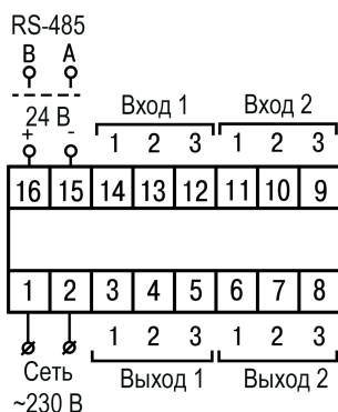
Рисунок 5.5 – Общая схема подключения TPM12–Щ5
