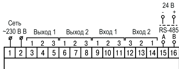
Рисунок 5.7 – Общая схема подключения TPM12–Н
