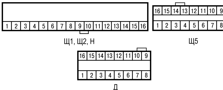
Рисунок 7.8 – Установка переключки
