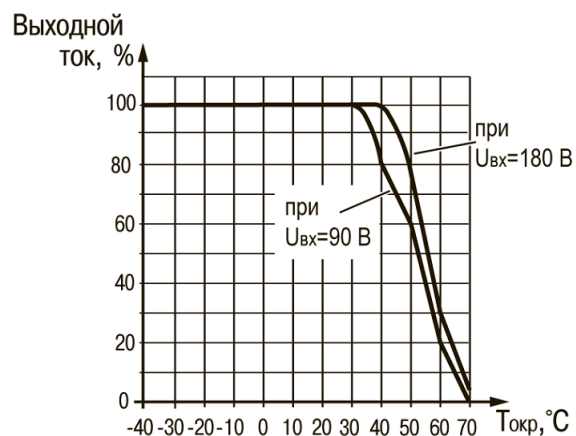
Рисунок 6.4 – График зависимости выходного тока ( U_{вых} = 24\text{ В} , режим Стенд) от температуры окружающей среды (дерейтинг)
