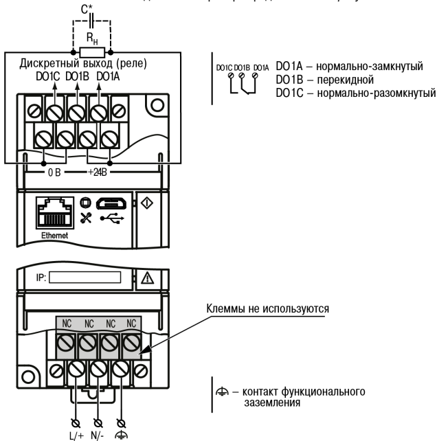
Рисунок 5 – Схема подключения
