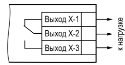
Рисунок 12 – Подключение нагрузки к ВУ типа «P»
