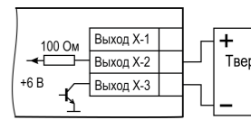
Рисунок 13 – Подключение нагрузки к ВУ типа «T»
