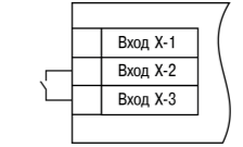
Рисунок 6 – Схема подключения к дискретному входу
