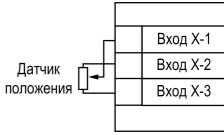
Рисунок 7 – Подключение датчика положения резистивного типа
