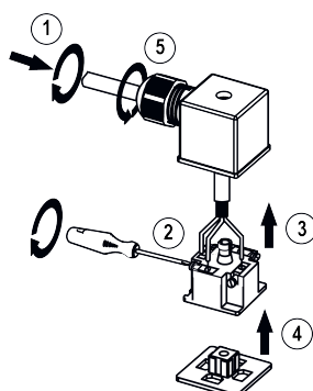
Рисунок 2 – Порядок подключения проводов ИП
