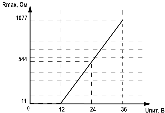
Рисунок 5 – График выбора допустимых значений сопротивления нагрузки
