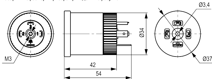
Рисунок 1 – Габаритные размеры прибора
