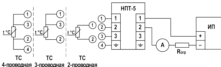
Рисунок 4 – Подключения прибора
