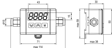
Рисунок 2 – Габаритные размеры корпуса НЗ
