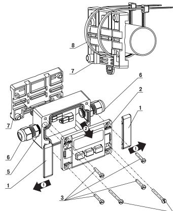
Рисунок 1 – Монтаж прибора
