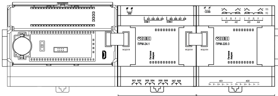
Рисунок 8 – Расположение модулей расширения на шине
