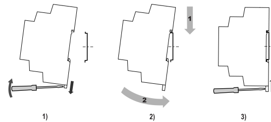
Рисунок 1 – Монтаж прибора
