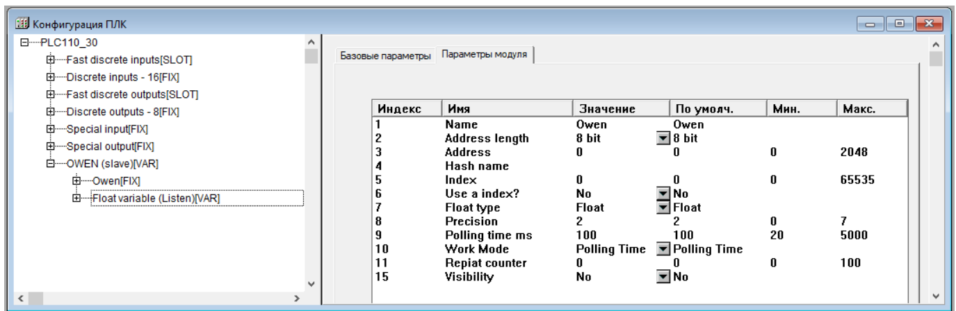
Рисунок 10.43 – Параметры переменных протокола ОВЕН
