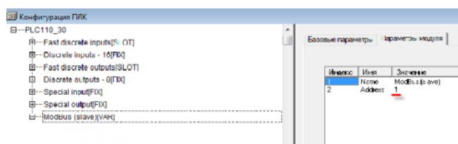
Рисунок 13.13 – Добавление и настройка элемента Modbus (Slave)
