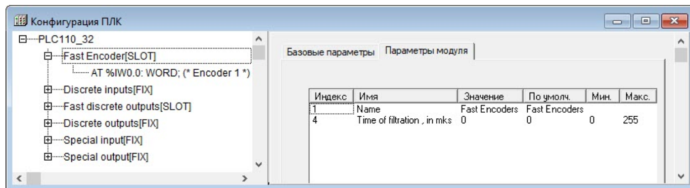
Рисунок 10.13 – Параметры модуля Высокочастотный энкодер (FastEncoder) для ПЛК110-32
