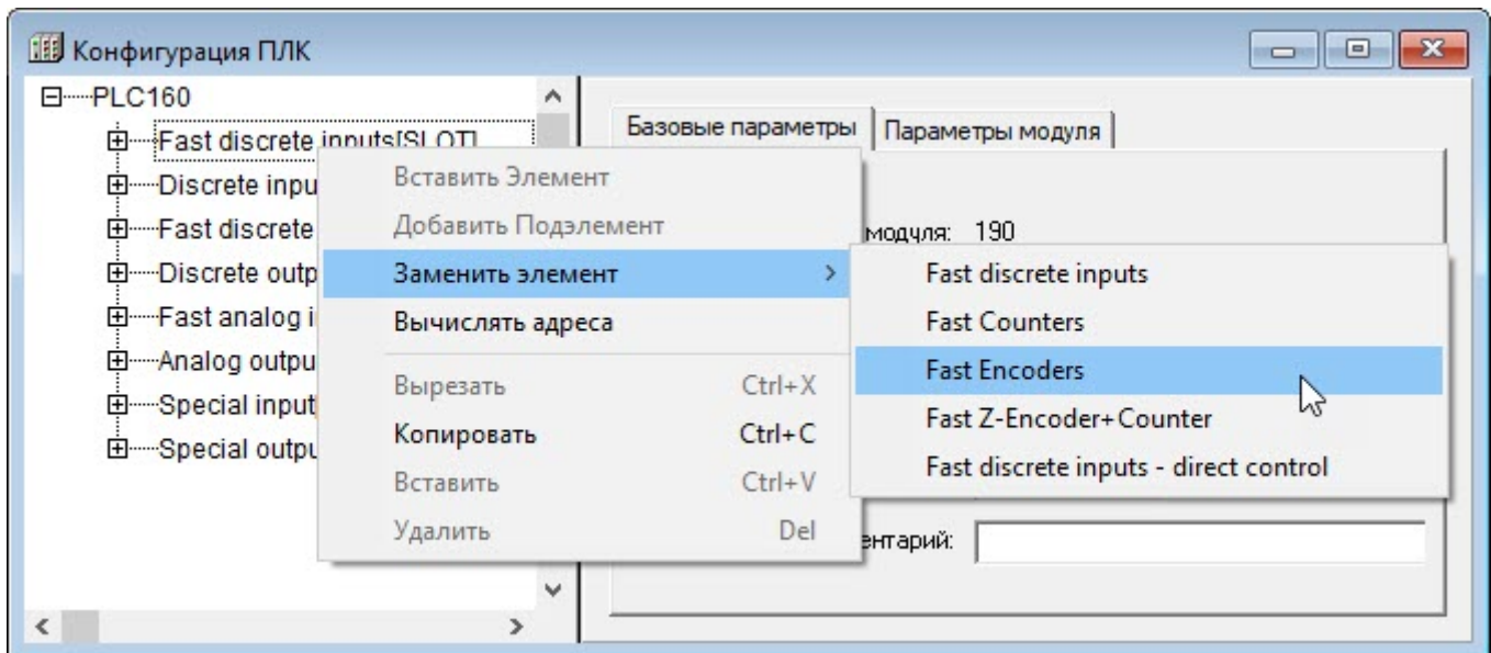
Рисунок 10.12 – Модули для замены модуля «Быстрые дискретные входы» (Fast discrete input)
