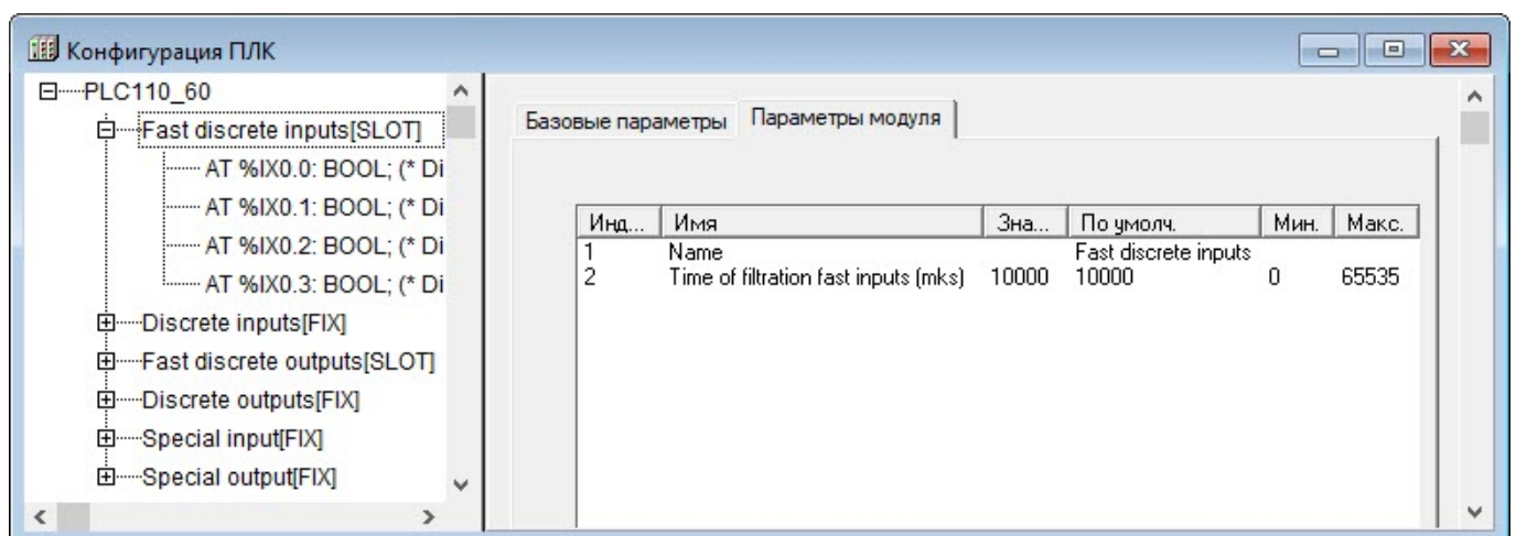
Рисунок 10.11 – Параметры модуля быстрых (высокочастотных) дискретных входов (Fast Discrete input)
