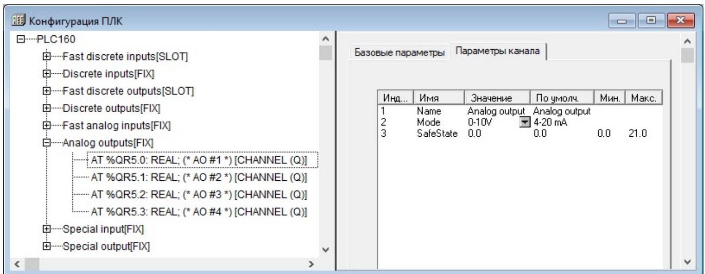
Рисунок 10.22 – Параметры модуля аналогового выхода
