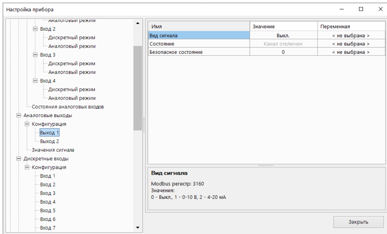
Рисунок 4.12 – Настройка универсальных аналоговых выходов
