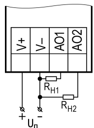
Рисунок 6.14 – Подключение аналогового выхода, находящегося в режиме источника напряжения
