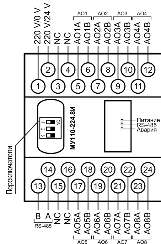
Рисунок 1 – Назначение контактов клеммника
