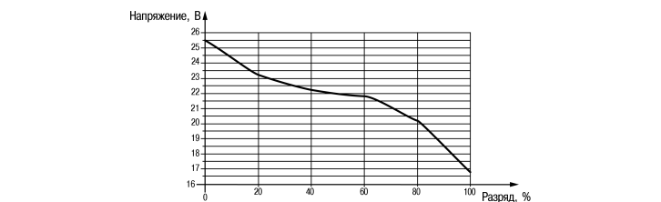
Рисунок 6.3 – График разряда током 3,6 А
