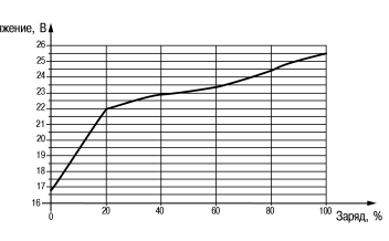
Рисунок 6.2 – График заряда током 0,8 А
