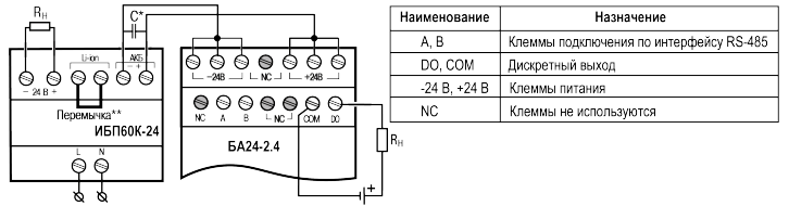
Рисунок 5.1 – Схема подключения
