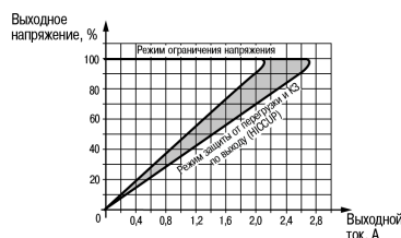
Рисунок 3 – График зависимости выходного напряжения от выходного тока (НИССУР)
