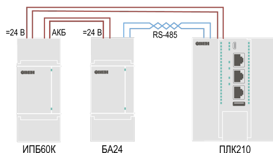
Рисунок 5.5 – Подключение к локальному Мастеру RS-485
