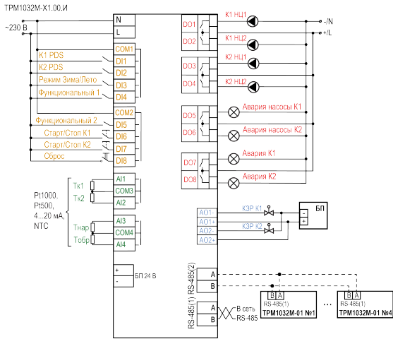
Рисунок 2 – Схема подключения
